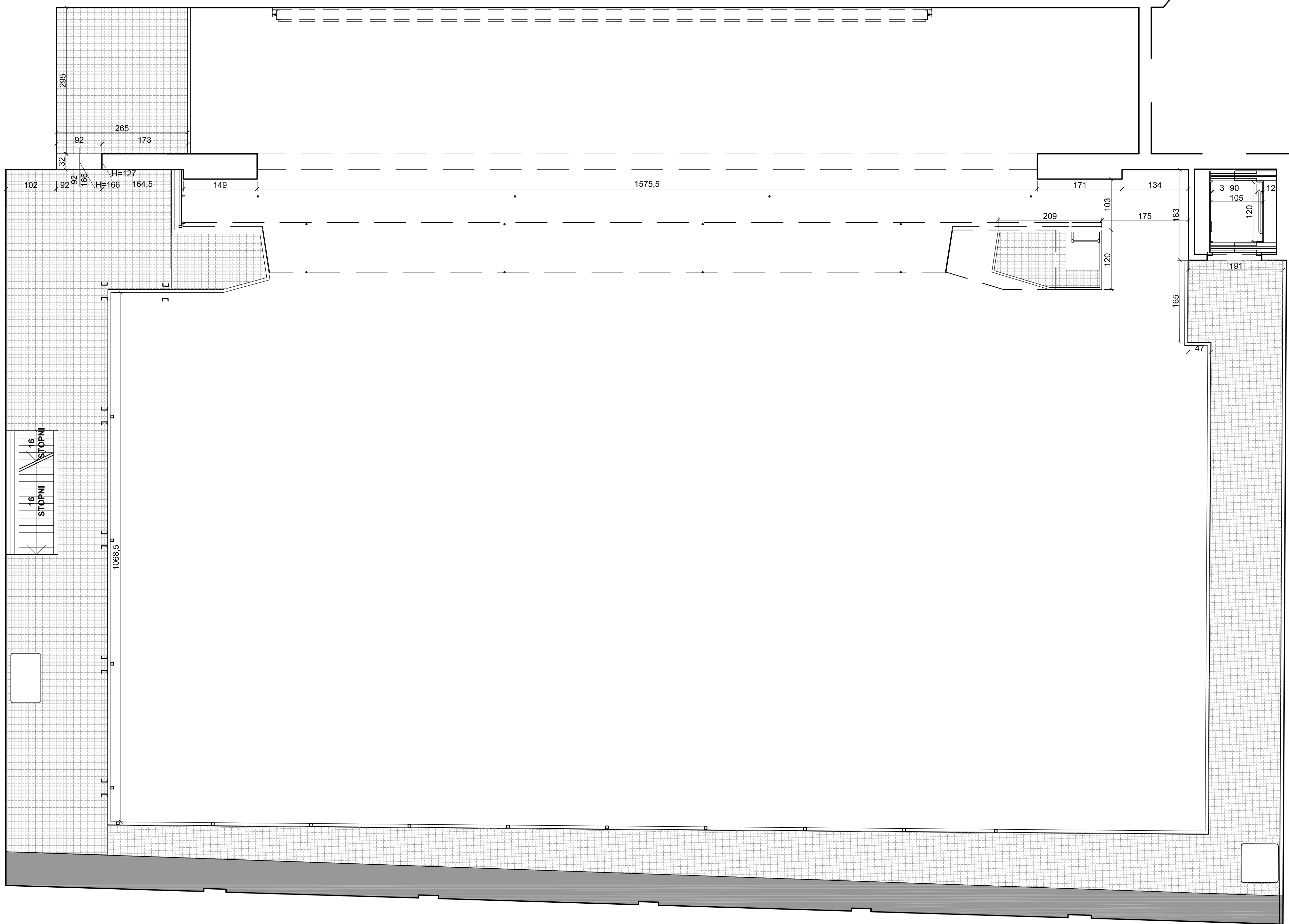
GALERIA TECHNICZNA - POZIOM +5,72/ II BALKON WIDOWNI skala 1:50
